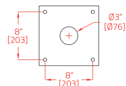
WXB-140 FOOTPRINT
