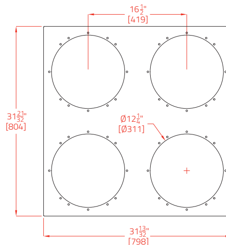
WXB-140 LID TOP VIEW
